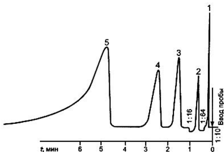
Типовая хроматограмма растворителя марки 645
